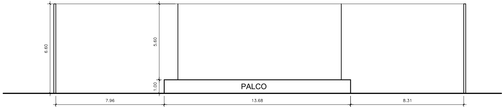
VISTA - BOCA DE PALCO - HÍPICA HALL SEM ESCALA
